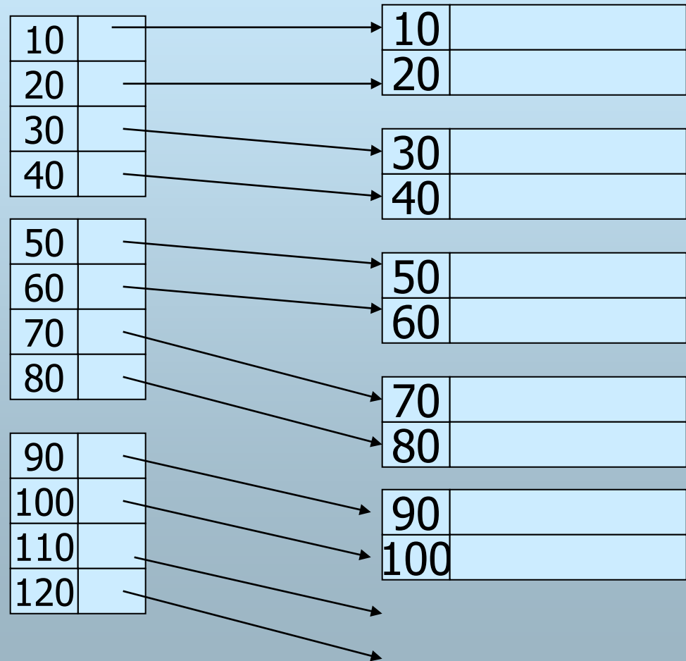
Dense Index
