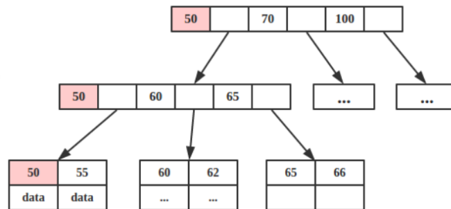
B+树
