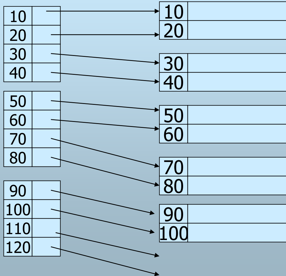
Dense Index
