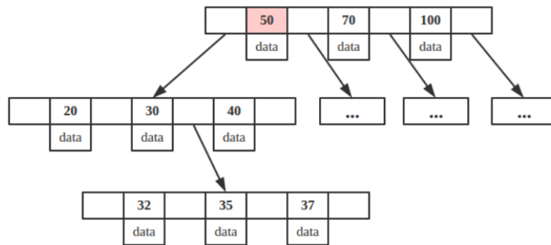
B-树
