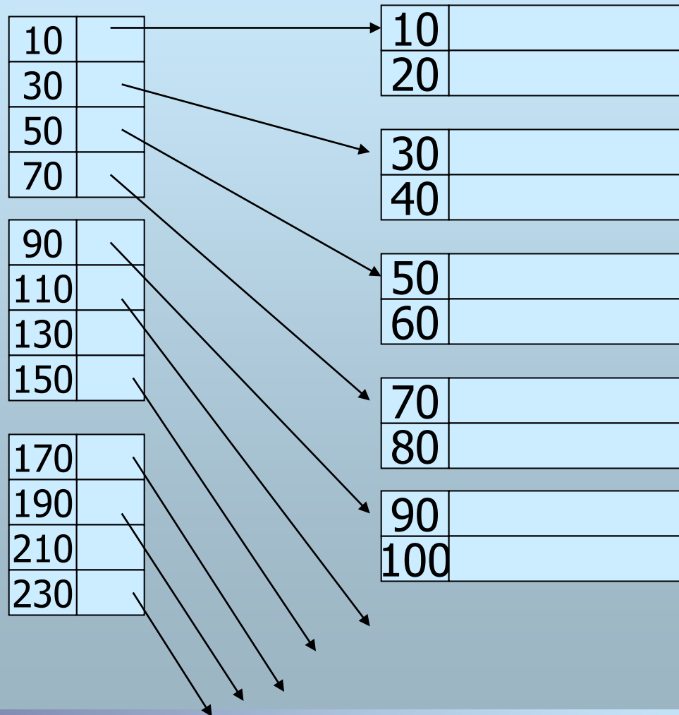
Sparse Index
